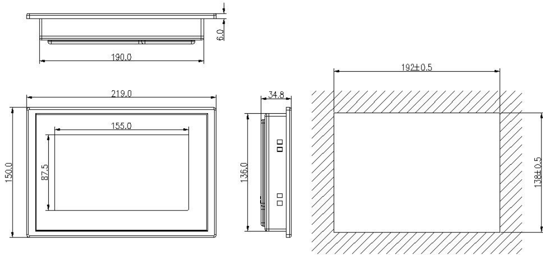
外形尺寸
